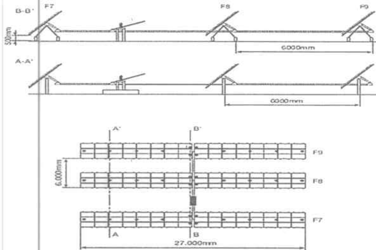
Figura N° 1 dimensiones de la estructura.
